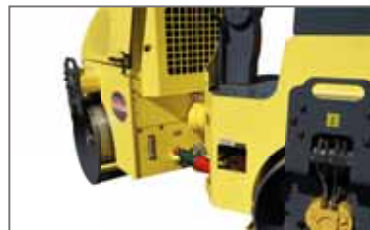
Double articulation avec points de graissage 'Pac-pivot' (breveté)
